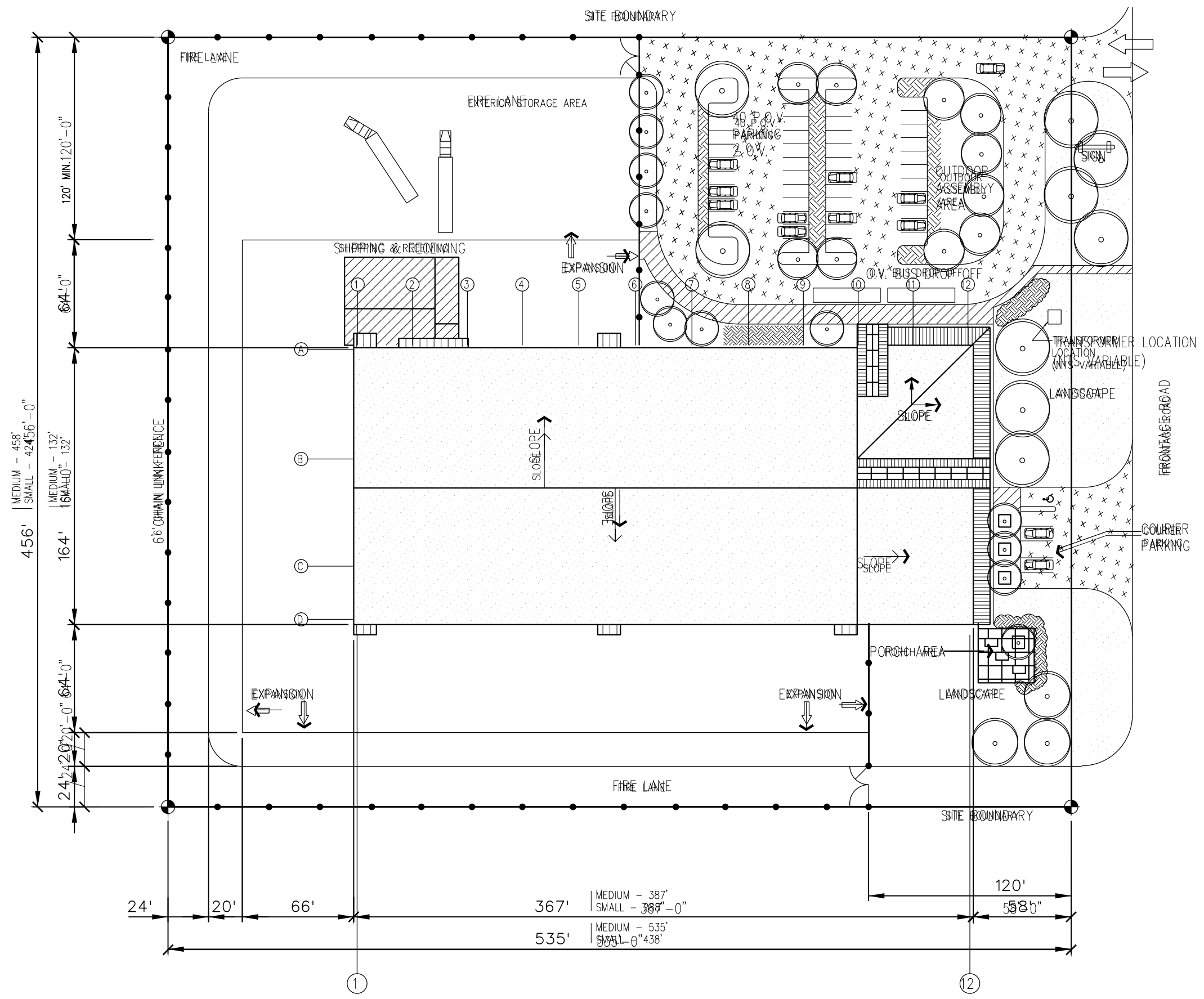
1 CENTRAL ISSUE FACILITY SITE LAYOUT (MEDIUM) SCALE: N.T.S.
